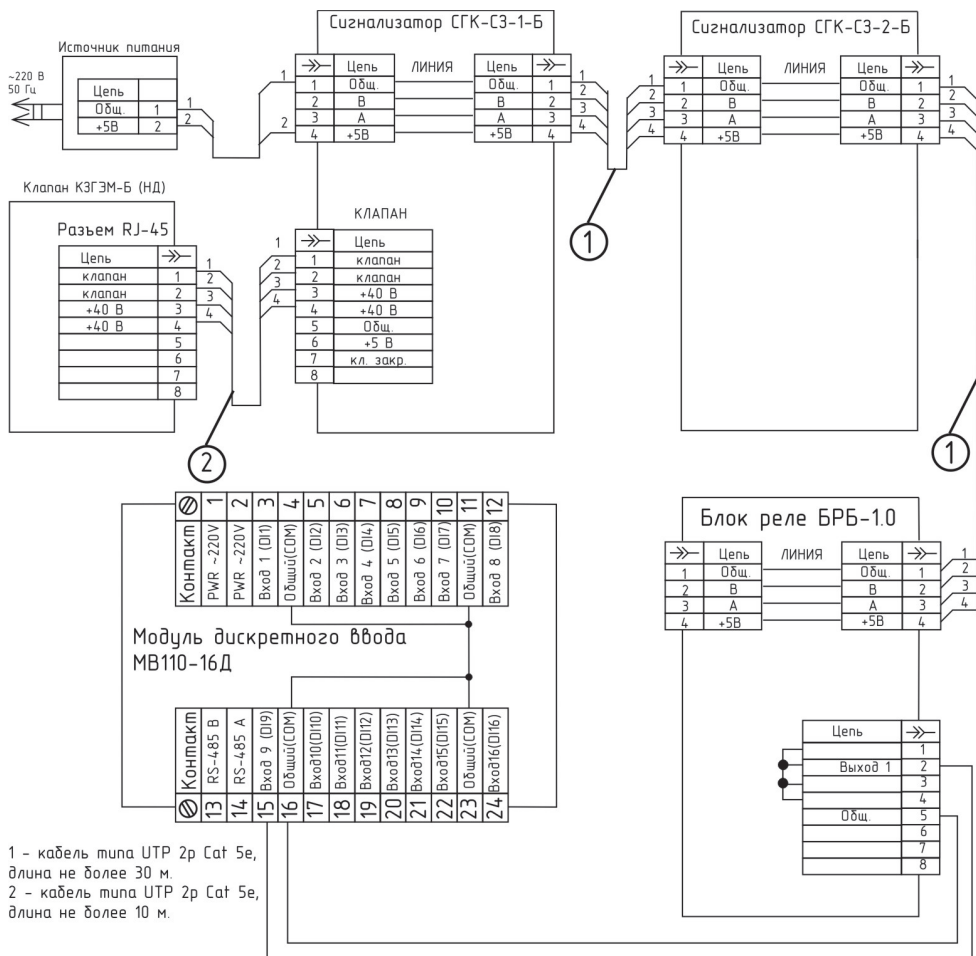
Рис. 2. Пример подключения системы автономного контроля загазованности с блоком реле БР-Б-1.0 к модулю дискретного ввода МВ110-16Д.
