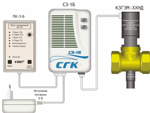
Рис. 2. Схема электрических соединений сигнализаторов СЗ-Б и бытового электромагнитного клапана КЗГЭМ-Б(без узла индикации положения клапана).
