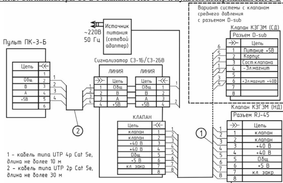
Рис.3. Сигнализаторы СЗ-Б с клапаном КЗГЭМ и пультом контроля ПК-3-Б
