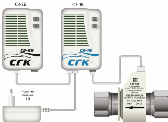
Рис. 4. Схема электрических соединений сигнализаторов СЗ-хБ, электромагнитного клапана КЗГЭМ и пульта контроля ПК-3-Б.
