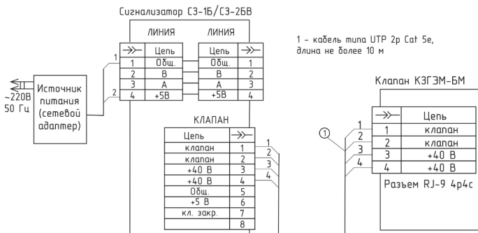
Рис. 2. Схема электрических соединений сигнализаторов СЗ-Б и бытового электромагнитного клапана КЗГЭМ-Б(без узла индикации положения клапана).
