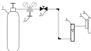
Рисунок Б.1 – Рекомендуемая схема подачи ГС на вход сигнализаторов загазованности бытовых СЗ-Б
