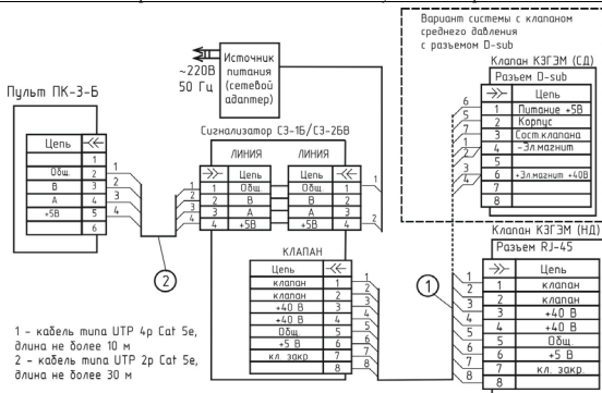
Рис.3. Сигнализаторы СЗ-Б с клапаном КЗГЭМ и пультом контрольным ПК-3-Б
