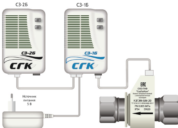
Рис. 5. – Система автономного контроля загазованности СГК-2-Б.
