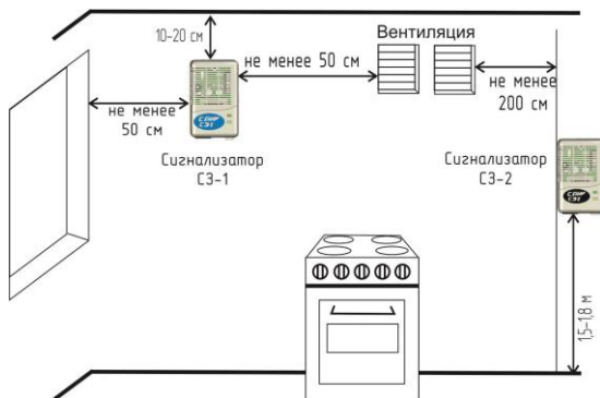
Рисунок 3 – Схема размещения сигнализаторов загазованности СГК СЗ-Х.
