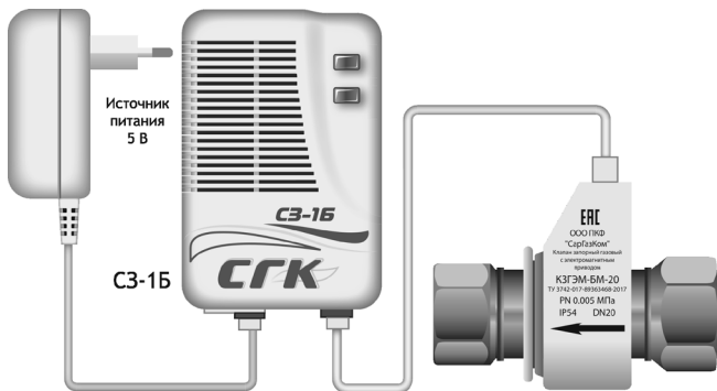
Рис. А1. Сигнализаторы загазованности бытовые С3-Б с клапаном типа КЗЭМ-БМ.
