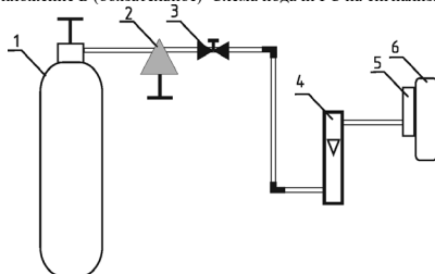
Приложение Б (обязательное) Схема подачи ГС на сигнализатор
