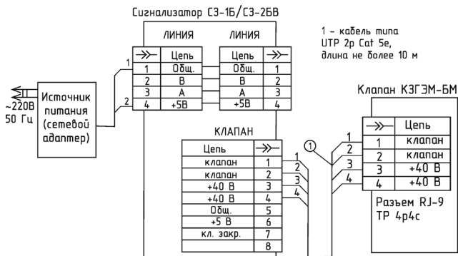
Рис. А2. Схема электрических соединений сигнализаторов С3-Б и бытового электромагнитного клапана КЗЭМ-Б(без узла индикации положения клапана).
