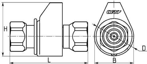
Рисунок 4. – Габаритные размеры клапана КЗГЭМ-Б.
