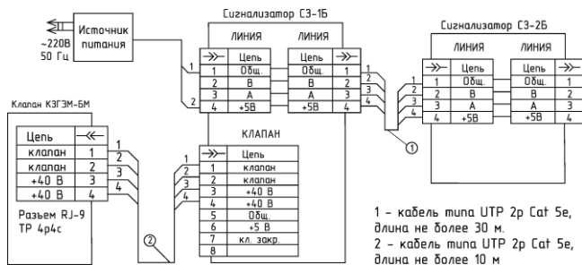
Рис. А6. – Система автономного контроля загазованности SGK-2Б. Схема электрических соединений
