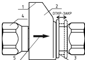
Рисунок 6. – Клапан КЗГЭМ-БМ
