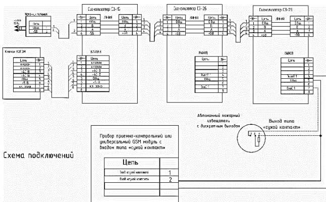
Рис.3. Пример подключения системы автономного контроля загазованности к модулю дискретного ввода MB110-16Д и пожарным извещателем
