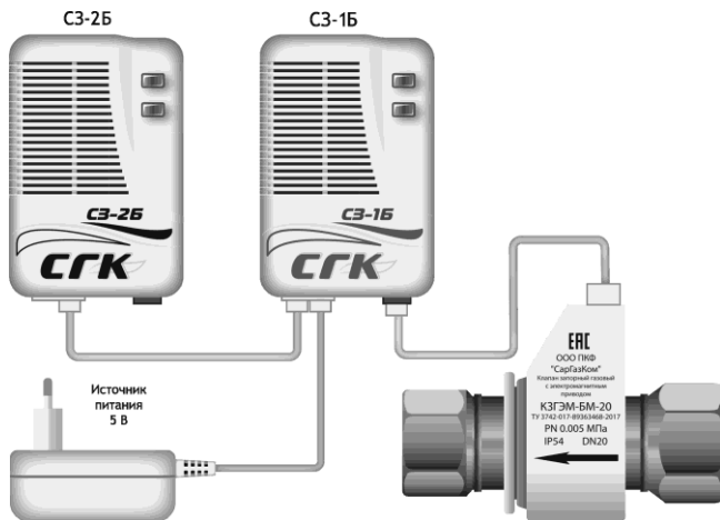
Рис. А5. – Система автономного контроля загазованности SGK-2Б
