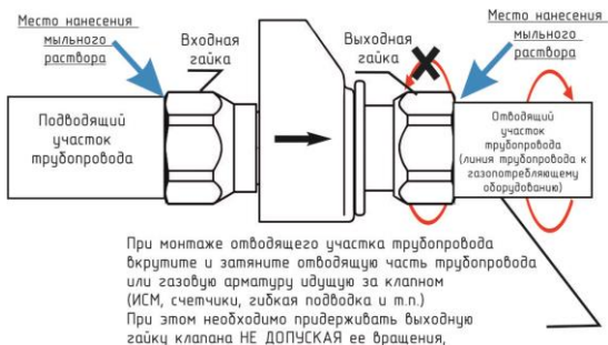
Схема 2. Порядок монтажа отводящего участка трубопровода к клапану
