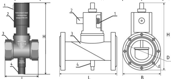
Рисунок 3. – Клапан КЗГЭМ.
