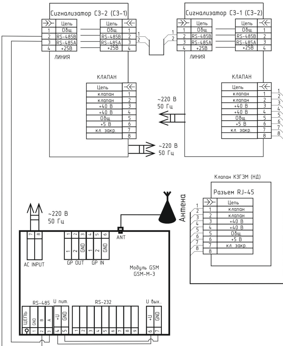
Рис 2. Схема подключения изделия к системе автономного контроля Загазованности СТК-2
