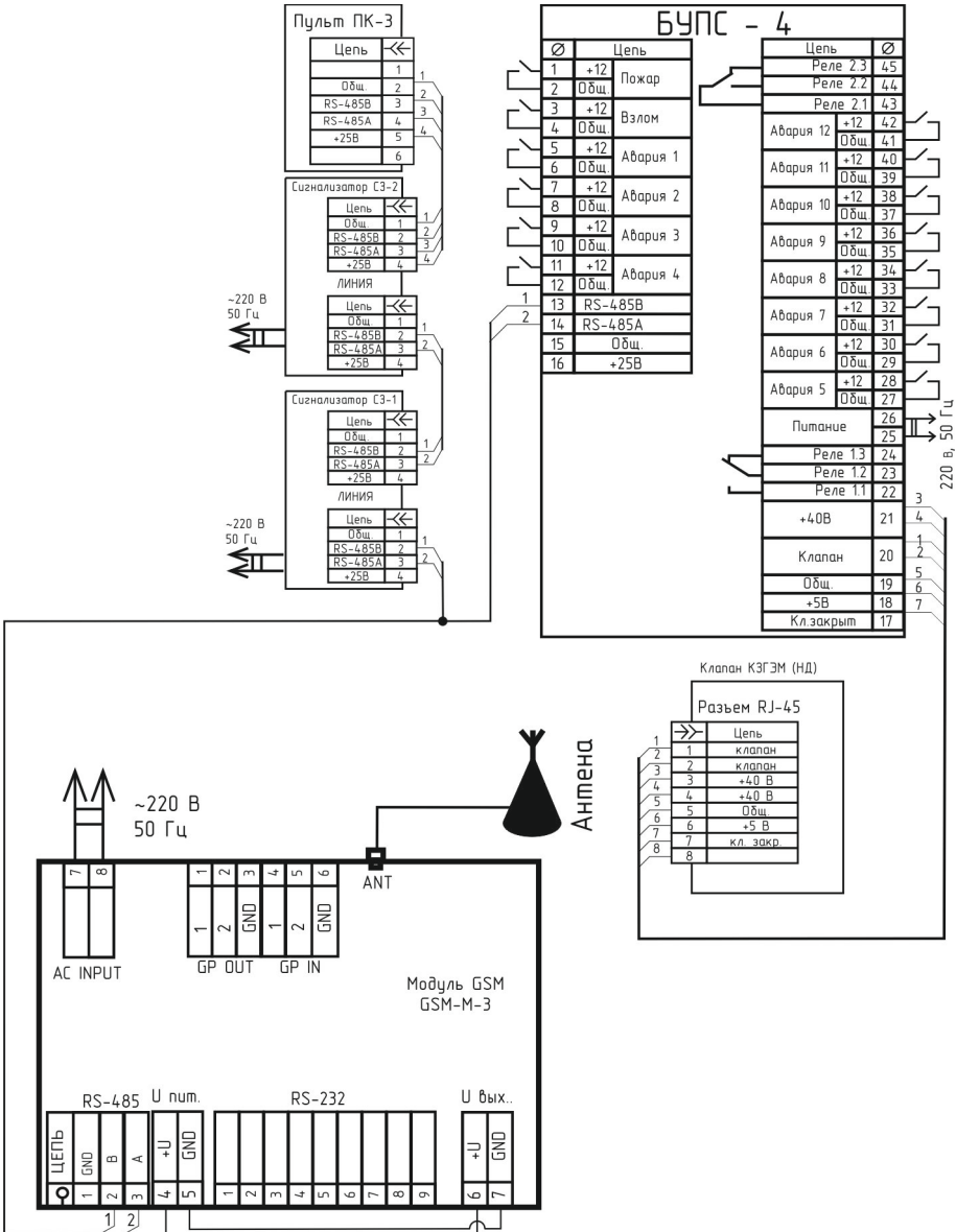
Рис 1. Схема подключения изделия к системе автономного контроля Загазованности СГК-3.
