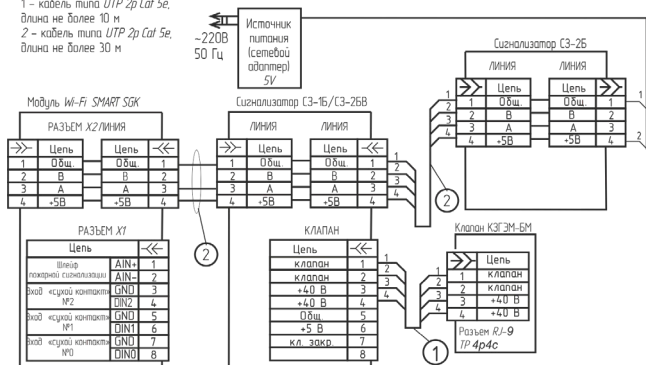
Рис. А5. – Система автономного контроля загазованности CGK-2-Б с Wi-Fi модулем SMART SGK
