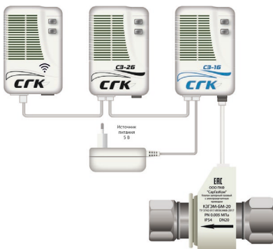
Рис. А5. – Система автономного контроля загазованности CGK-2-Б с Wi-Fi модулем SMART SGK
