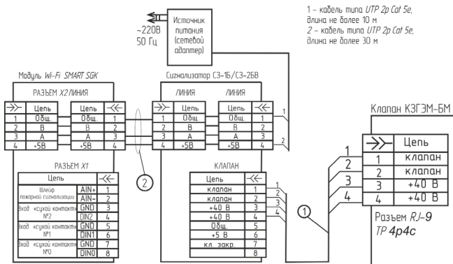
Рис. А2. Схема электрических соединений сигнализаторов C3-хБ, электромагнитного клапана КЗЭМ-БМ и Wi-Fi модуля SMART SGK.
