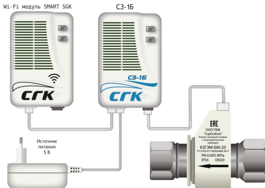
Рис. А1. Сигнализаторы C3-Б с клапаном КЗЭМ-БМ и Wi-Fi модулем SMART SGK.
