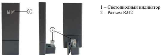
Рисунок 1. – Модуль. Внешний вид.
